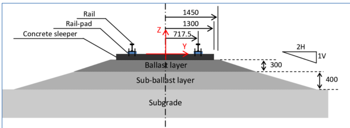
Figura 2.1_Prerje tërthore e trasesë së hekurudhës
